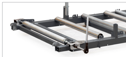
Drivpaket på lastbäraren som underlättar inlastningen
