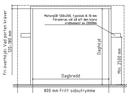
Sidomonterat motorspel
