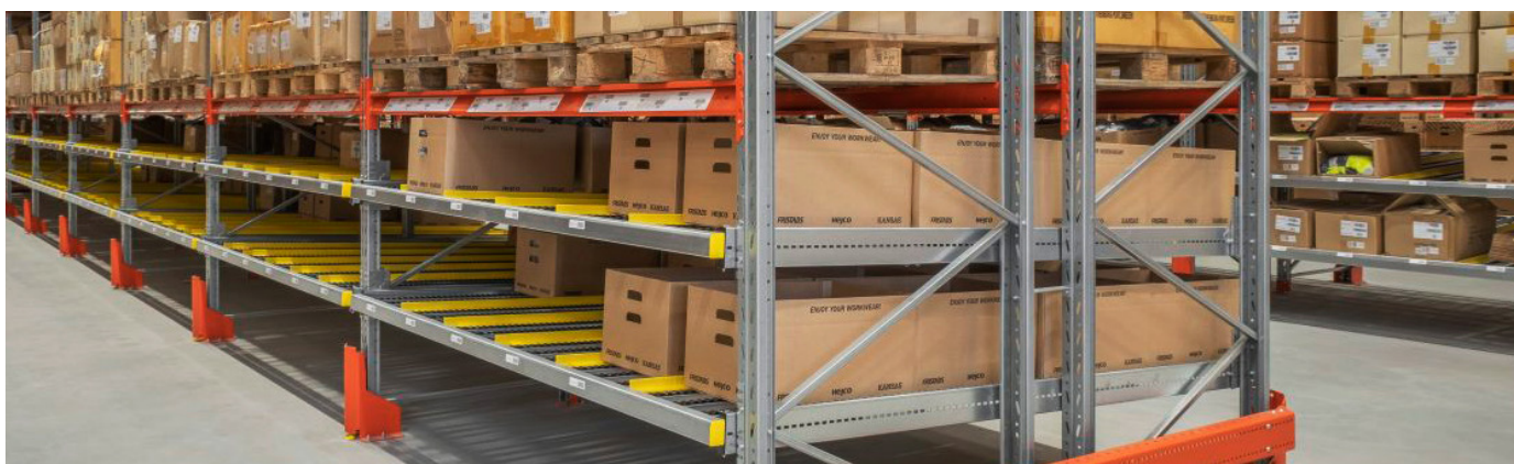
Carton Flow för plockgoods, monterade i pallställ Omega.
