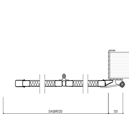
Övermonterat motorspel med arm för begränsat sidoutrymme
