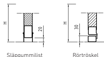
Släpgummlist
