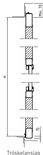
Tröskelanslag
