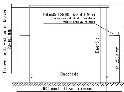
Sidomonterat motorspel
