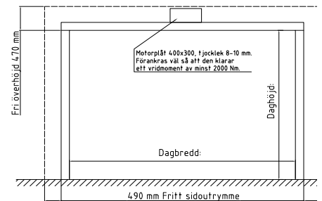
Övermonterat motorspel, standard montage
