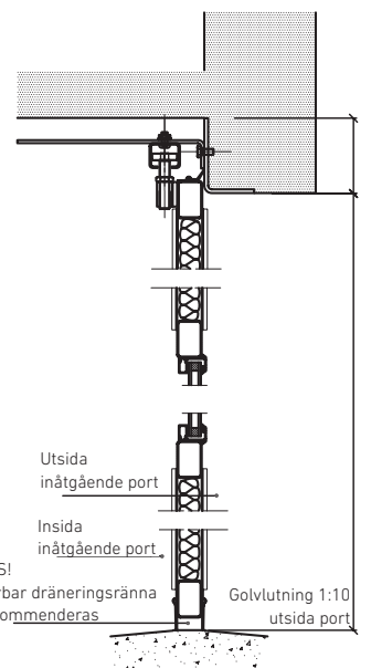
Styrbeslag
