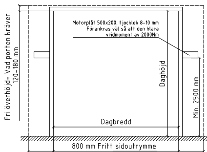
Sidmonterat motorspel
