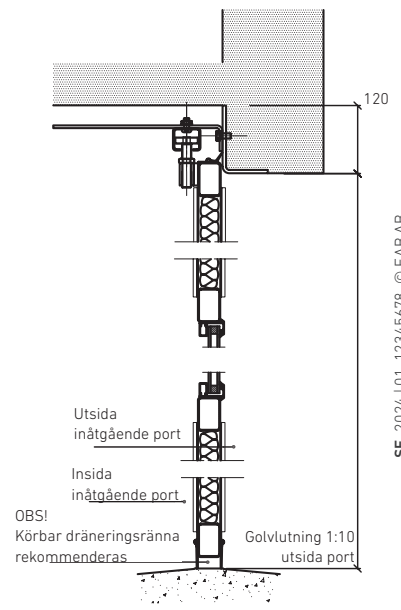
Styrbeslag
