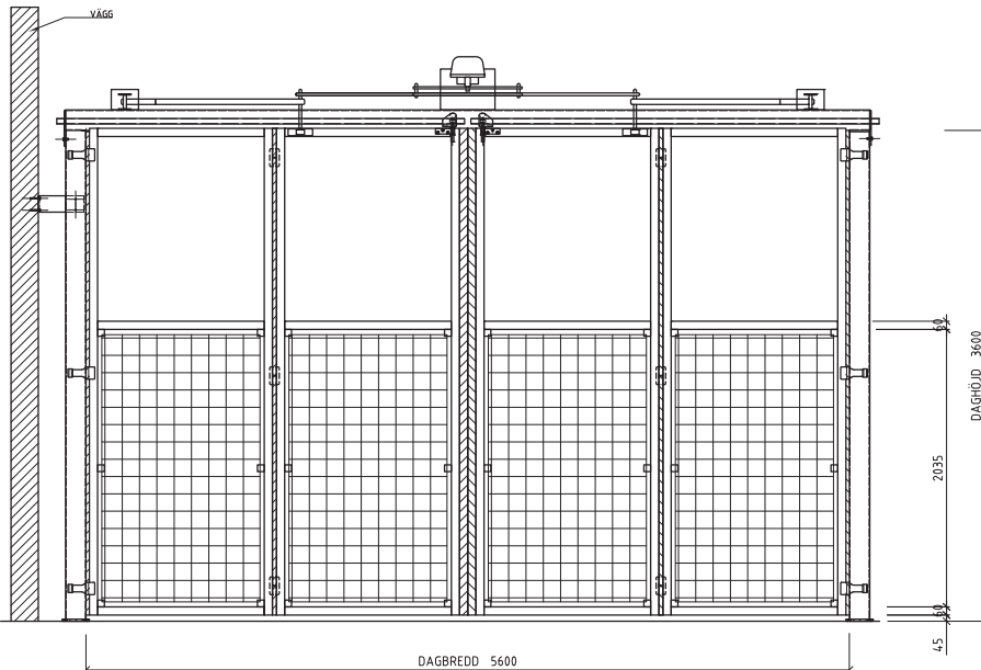
4-DELAD VIKPORT MED EL-DRIFT SEDD FRÅN MASKINSIDAN
