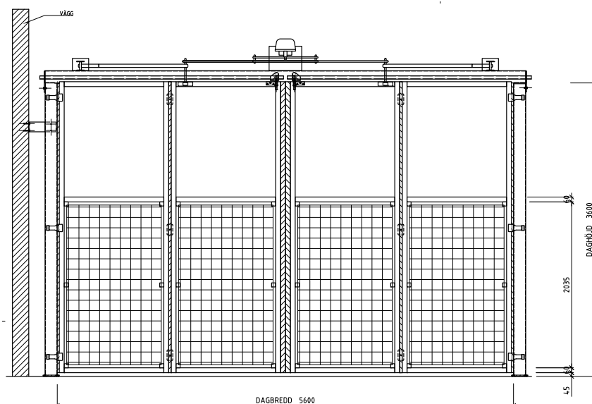
4-delad vikport med el-drift, sedd från maskinsidan.
