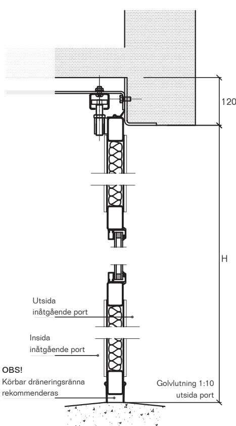
Styrbeslag Upp till 4,5 m portbredd
