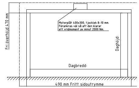
Övermonterat motorspel, standard montage
