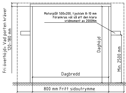
Sidomonterat motorspel
