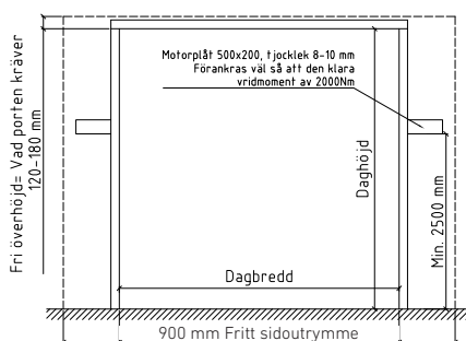
Sidomonterat motorspel
