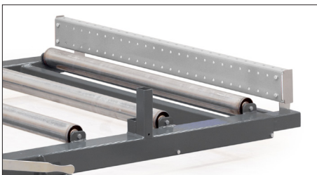
Stopp i bakkant på lastbäraren
