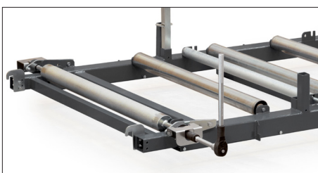
Drivpaket på lastbäraren som underlättar inlastningen
